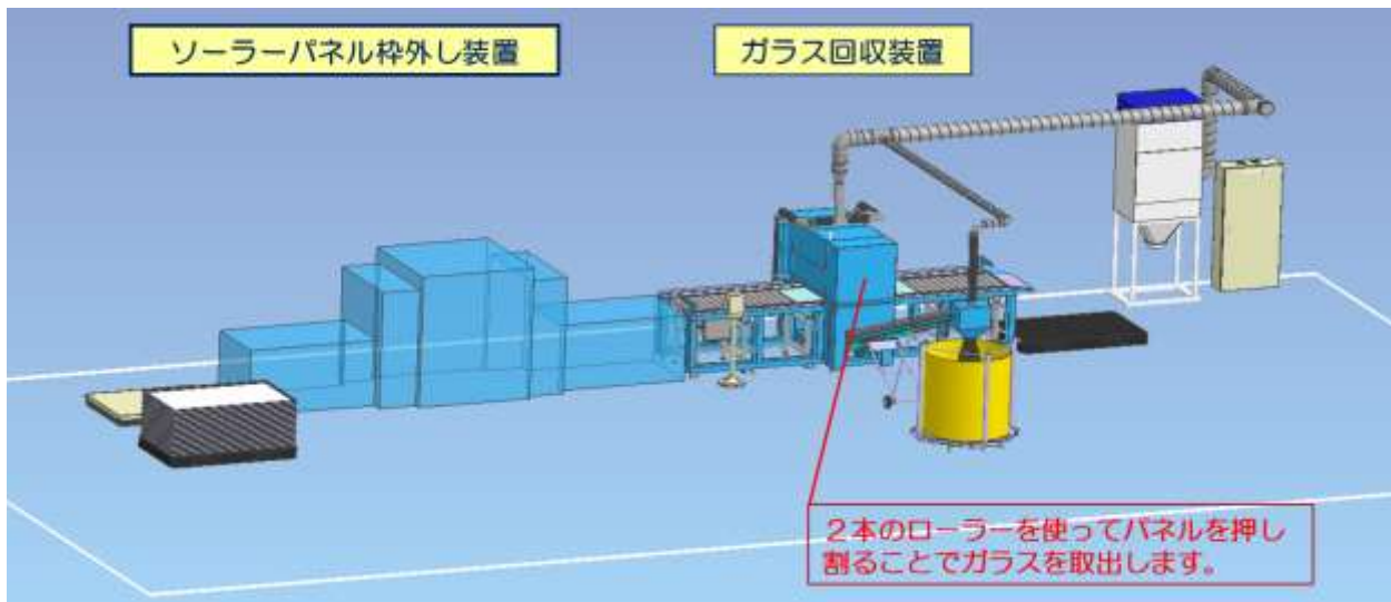
【共栄九州製太陽光パネルリサイクル装置】
